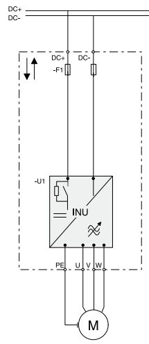
INU Inverter Unit (FR4-FR8)
